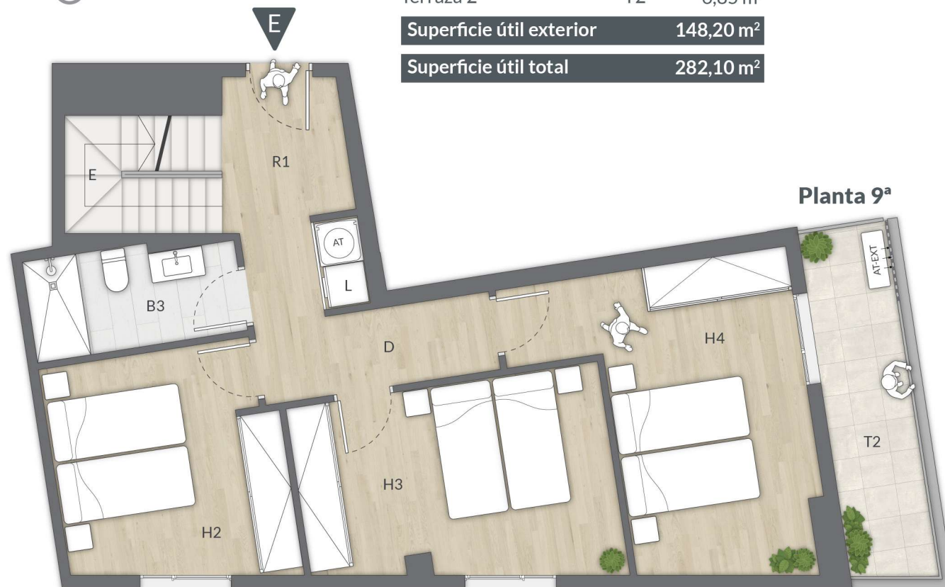
Planta Ático
